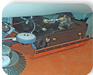
particolare della versione rulli
